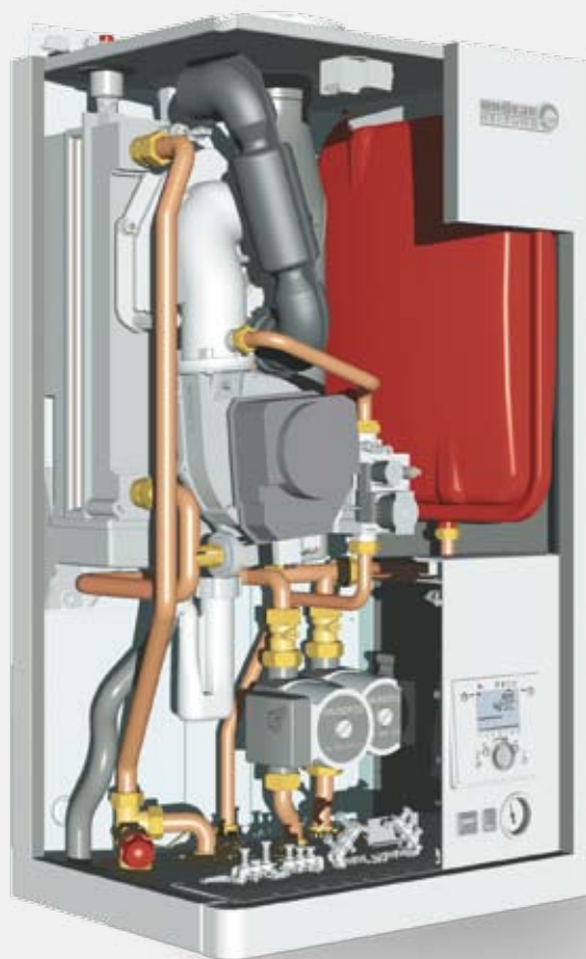
EcoTherm Plus WGB 15 C včetně příslušenství
